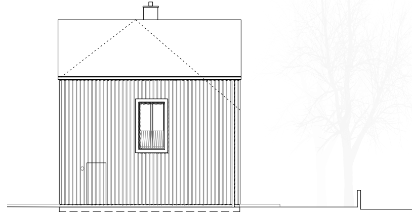
Ansicht Ost
