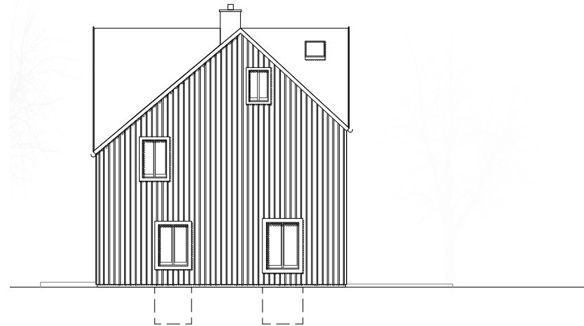
Ansicht West
