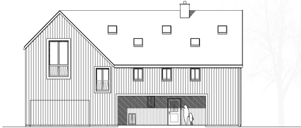
Ansicht Nord
